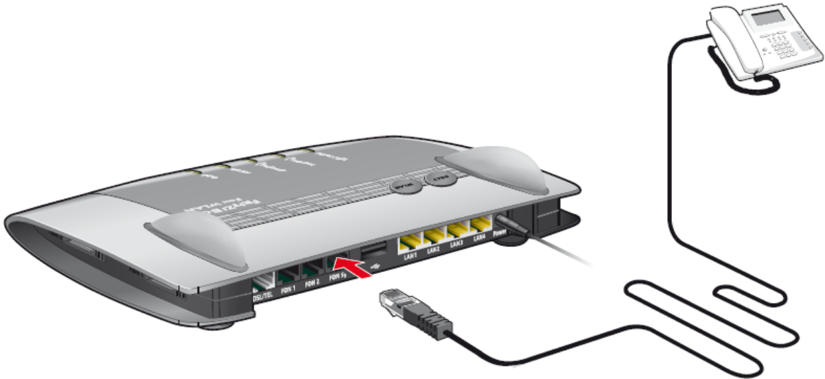
Anschluss von ISDN Geräten
