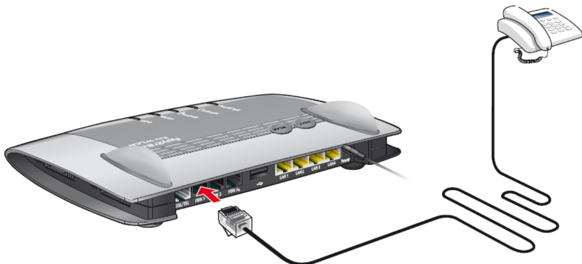
Anschluss eines Telefons mit RJ11 Stecker
