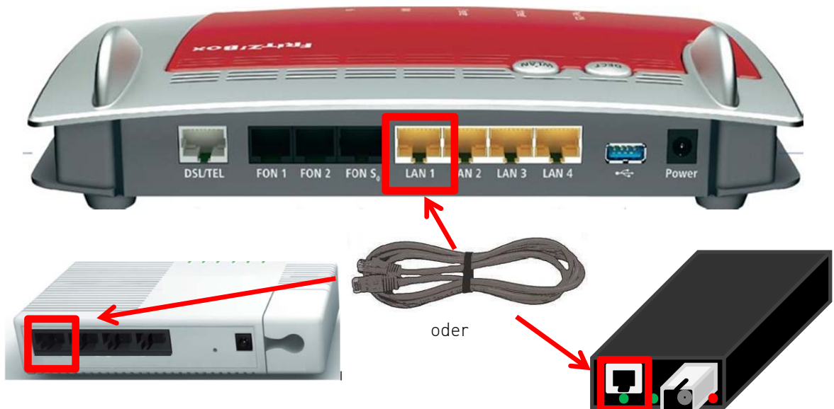
Anschließen des Glasfaser-Konverters
